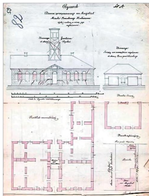
Ryc. 12. A. Borkowski-Dunin, Projekt przebudowy tzw. Domu Miejskiego w Hrubieszowie na ratusz (wraz z dodaniem mu wieży), 1844 (?), APL, RGL (1837–1866), oraz W. Konkowski, Pomiar inwentaryzacyjny tzw. Domu Miejskiego w Hrubieszowie, przebudowywanego według projektu A. Borkowskiego-Dunina na ratusz, 1847, APL, RGL (1837–1866), Adm. sygn. 476, k. 21 i 59. Fot. Pracownia Reprograficzna APL, [w:] J. Żywicki, op. cit. , ilustracja 18 i 19.
